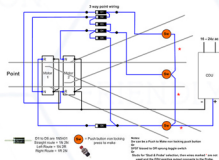
Point Wiring
